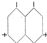
Chromotropsäure. D.R.P. 67563.
